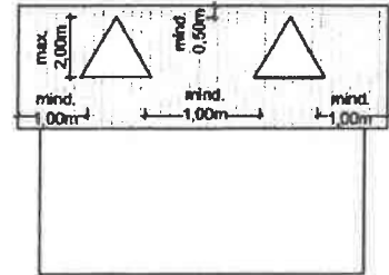
Dreiecksgaube
