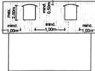
Segmentbogengaube
