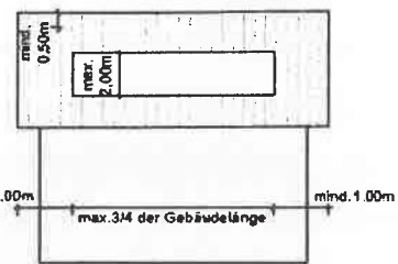
Flachdachgaube
